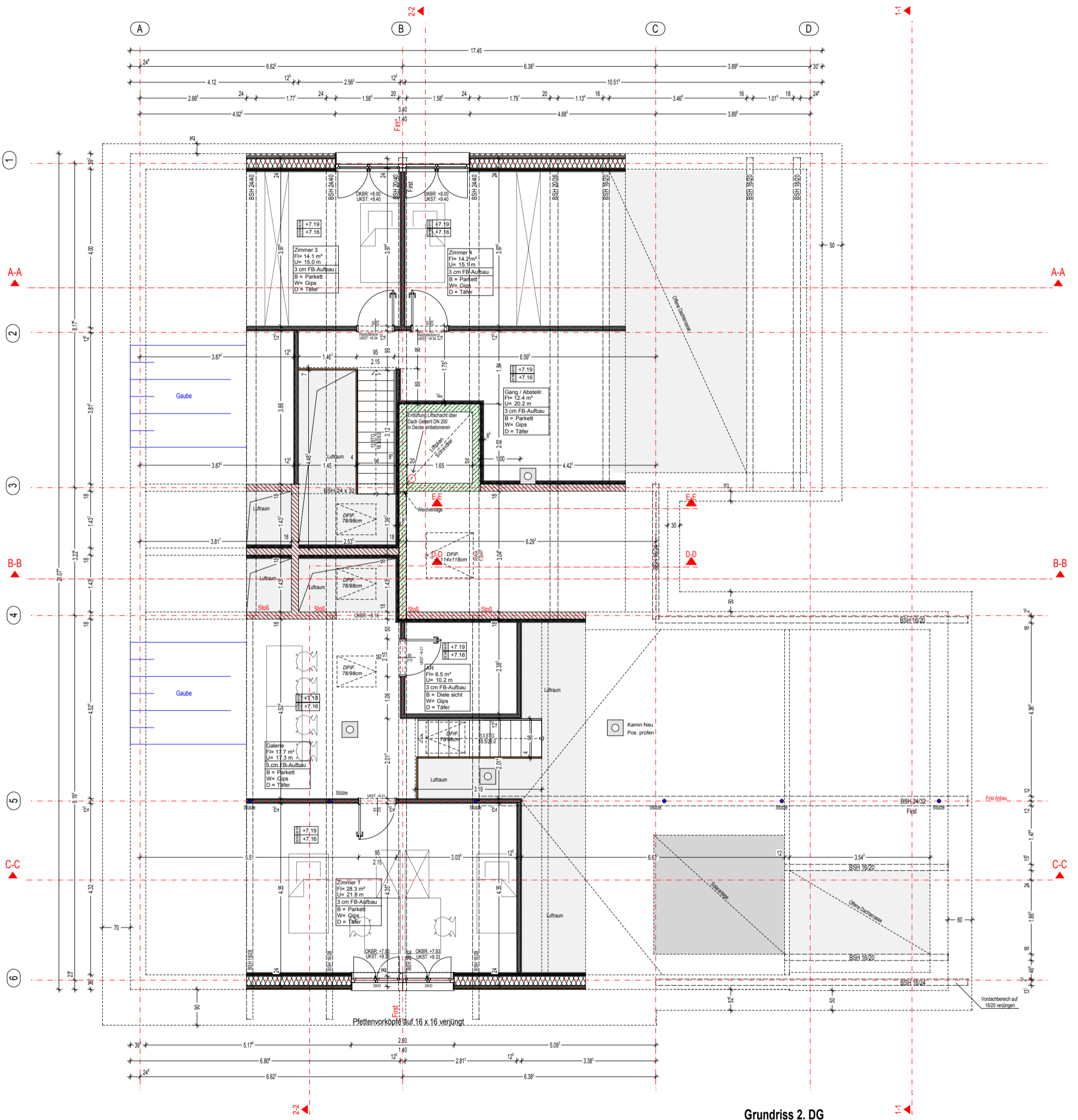
Grundriss 2. DG
